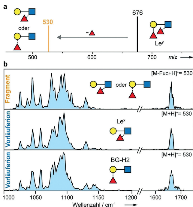
Abbildung 3. a) Schematisches Tandem-MS-Spektrum des \text{Le}^y -Tetrasaccharids als [\text{M}+\text{H}]^+ -Spezies. Das Hauptfragment ( m/z = 530 ) resultiert aus dem neutralen Verlust einer Fucoseeinheit. Das experimentelle Massenspektrum ist in den Hintergrundinformationen gezeigt. b) IR-Spektren des [\text{Le}^y\text{-Fuc}+\text{H}]^+ -Fragments sowie der intakten Standards \text{Le}^x und BG-H2 ( m/z = 530 ).
