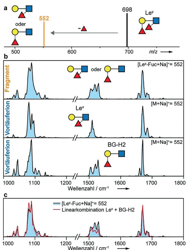
Abbildung 2. a) Schematisches Tandem-MS-Spektrum des Le y -Tetrasaccharids als [\text{M}+\text{Na}]^+ -Spezies. Das Hauptfragment ( m/z = 552 ) resultiert aus dem neutralen Verlust einer Fucoseinheit. Das experimentelle Massenspektrum ist in den Hintergrundinformationen gezeigt. b) IR-Spektren des [\text{Le}^y\text{-Fuc}+\text{Na}]^+ -Fragments und der intakten Standards Le x und BG-H2 ( m/z = 552 ). c) Das IR-Spektrum des Le y -Fragments als Natriumaddukt kann durch eine Linearkombination der individuellen Trisaccharidspektren von Le x und BG-H2 dargestellt werden.
